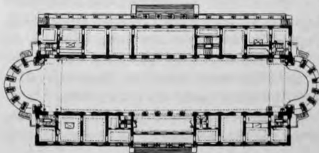
Дворец Г.А. Потёмкина в Осиновой Роще. Проект И.Е. Старова.
